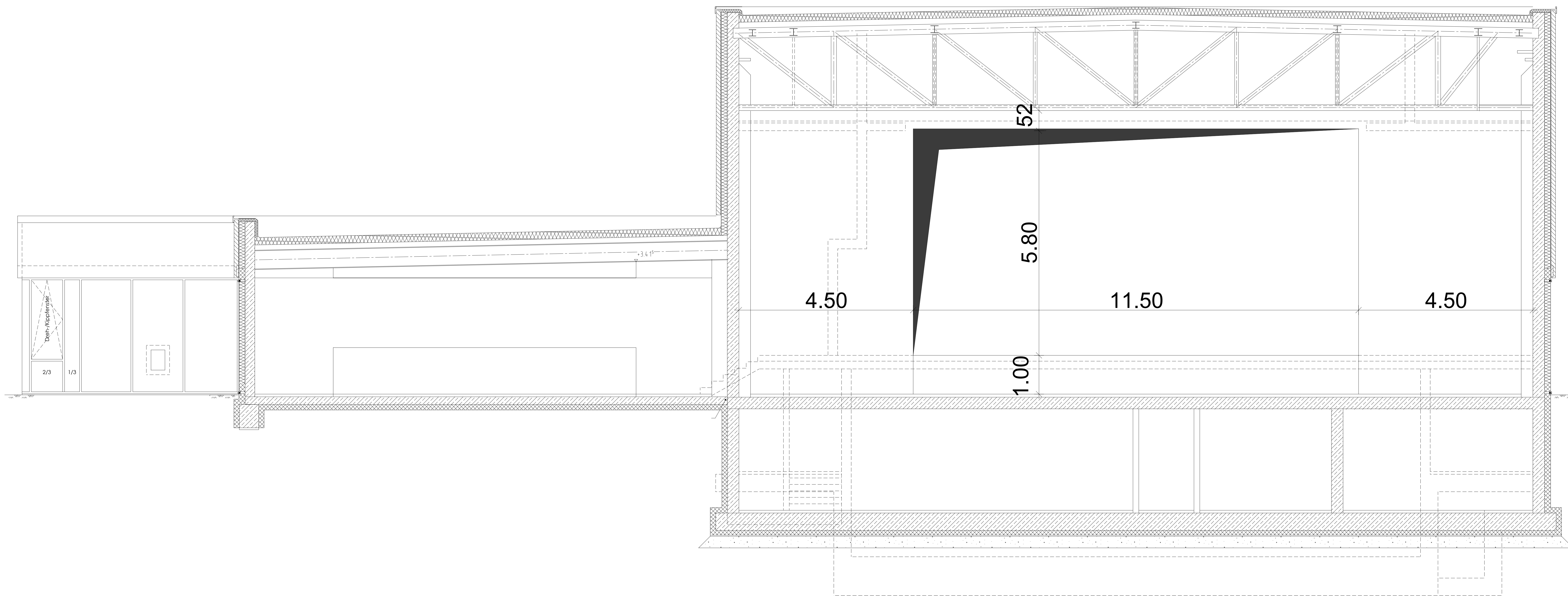
SCHNITT C-C
